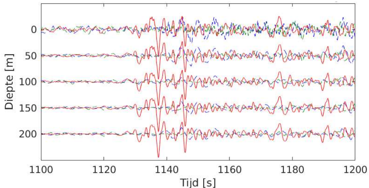
Figuur 2: Meting van de Papoea Nieuw Guinea 22-01-2017 beving op station G29 te Overschild. De beving heeft een magnitude van 7.9 en ligt op een epicentrale afstand van zo'n 14000 km. De grondbewegingen worden getoond op verschillende dieptes tussen 1100 en 1200 seconden na de aardbeving. Doorgetrokken lijnen geven verticale bewegingen weer, gestreepte lijnen horizontale bewegingen.
