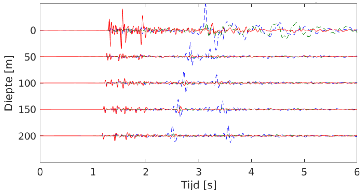
Figuur 1: Meting van de Wirdum 1-11-2016 beving op station G29 in Overschild. De beving heeft een magnitude van 2,2 en ligt op een epicentrale afstand van zo'n 3 km. De grondbewegingen worden getoond op verschillende dieptes, van 0 tot 6 seconden na de aardbeving. Doorgetrokken lijnen geven verticale bewegingen weer, gestreepte lijnen horizontale bewegingen.
